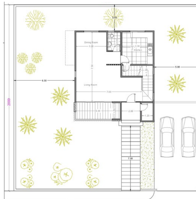
REZ-DE-CHAUSSÉE
