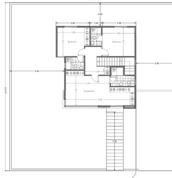
1 ER ETAGE
